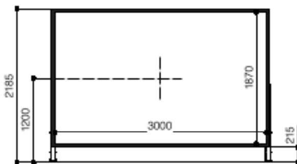
ZEN SCREEN 300x187 (pieds au sol en extension minimale)
