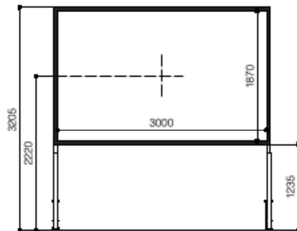
ZEN SCREEN 300x187 (pieds au sol en extension minimale)
