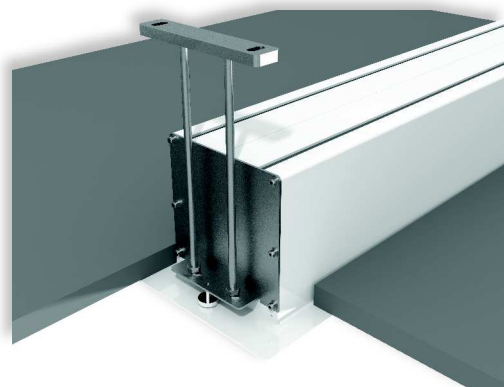
VUE DU COTE GAUCHE
